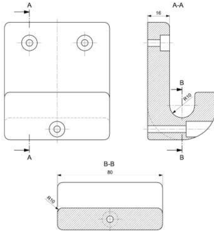
شکل ۸- قلاب آویز
